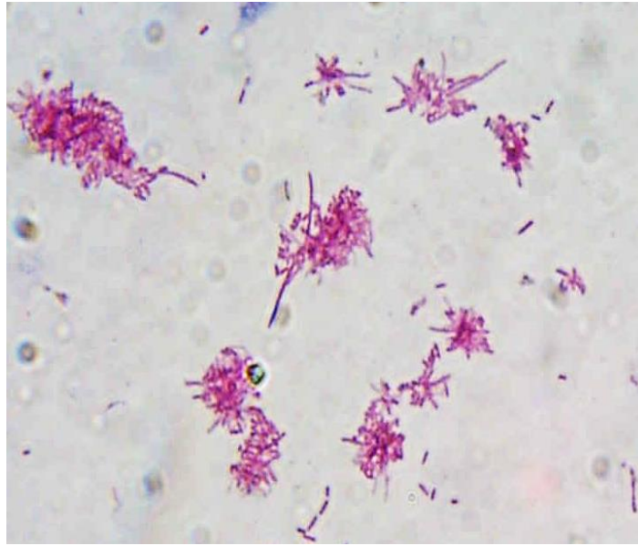
Slika 4.17. Mikrofotografija bakterijske kulture P. putide u 24. satu u P2 za kontrolu snimljena u prolaznoj svjetlosti, P = 1000 \times .
