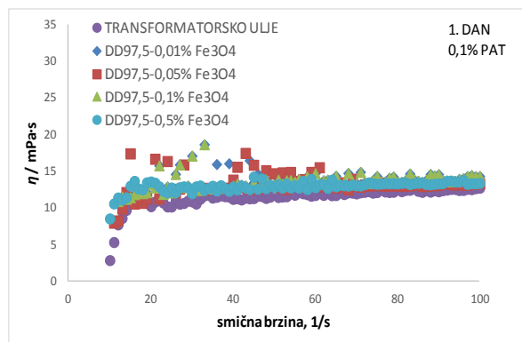
Slika 4.4.4.5. Ovisnost dinamičke viskoznosti o smičnoj brzini za transformatorsko ulje i uzorke s 0,1 mas. % PAT i različitim masenim udjelima Fe 3 O 4 nanočestica (1. dan)
