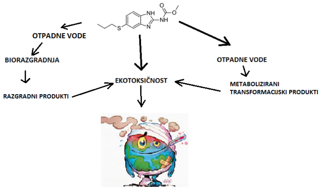
Slika 1. Sudbina antihelmintika albendazola u okolišu
