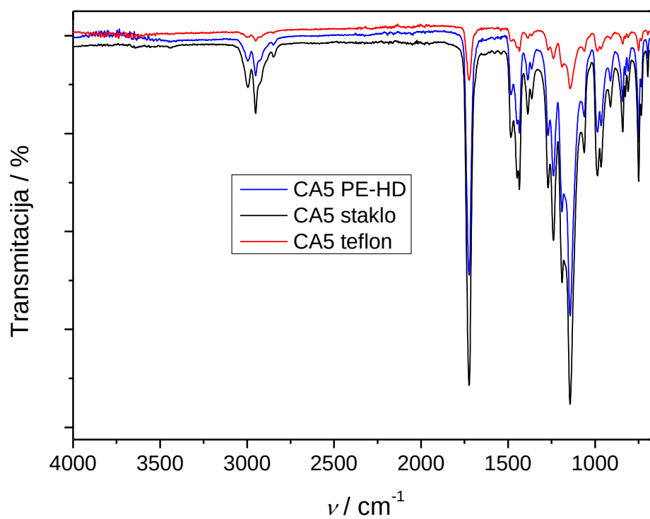
Slika 4.2.5 Infracrveni spekter za uzorak CA5 pripremljen na različitim podlogama
