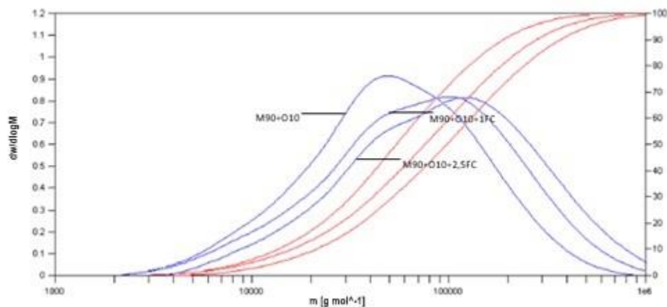
Slika 4.1.7. Raspodjele molekulskih masa neprešanih kompozita M90+10O s različitim udjelima FC
