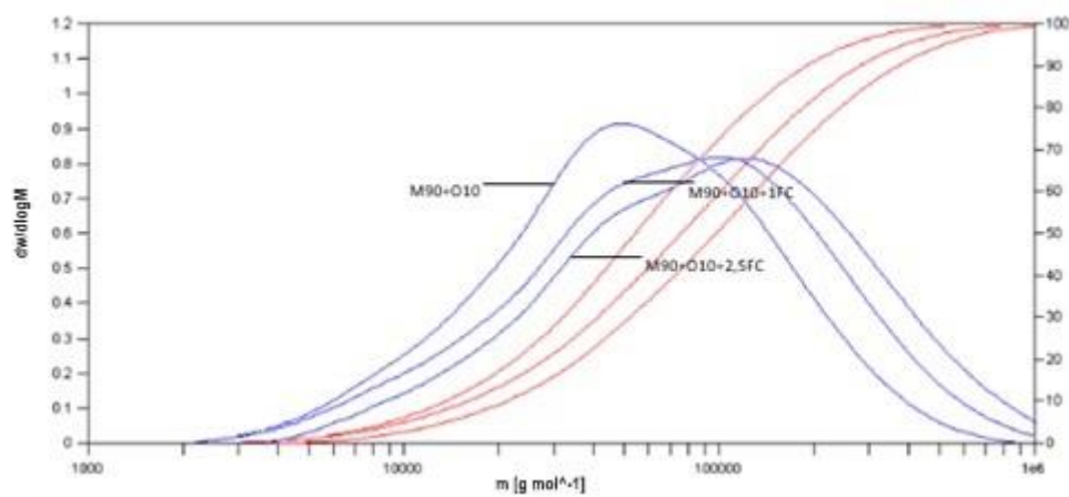
Slika 4.1.7. Raspodjele molekularnih masa neprešanih kompozita M90+100 s različitim udjelima FC
