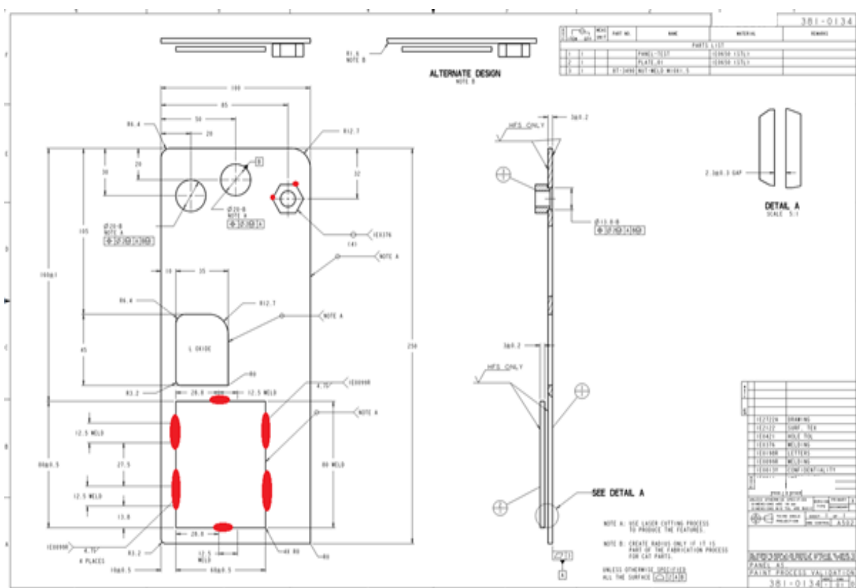
Slika 17.: Nacrt uzoraka na kojima su se izvodila ispitivanja (crveno označena mjesta varova)
