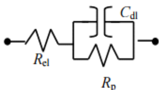
Slika 10.: Prikaz Randlesovog ekvivalentnog električni kruga [12]
