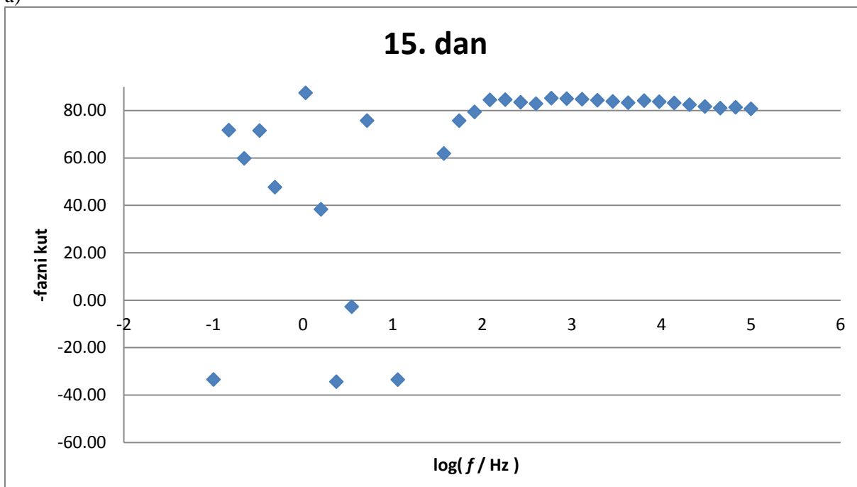
Slika 23.: Eksperimentalni podaci za EIS za 15. dan: a) ovisnost logaritma apsolutne impedancije o logaritmu frekvencije, b) ovisnost faznog kuta o logaritmu frekvencije
