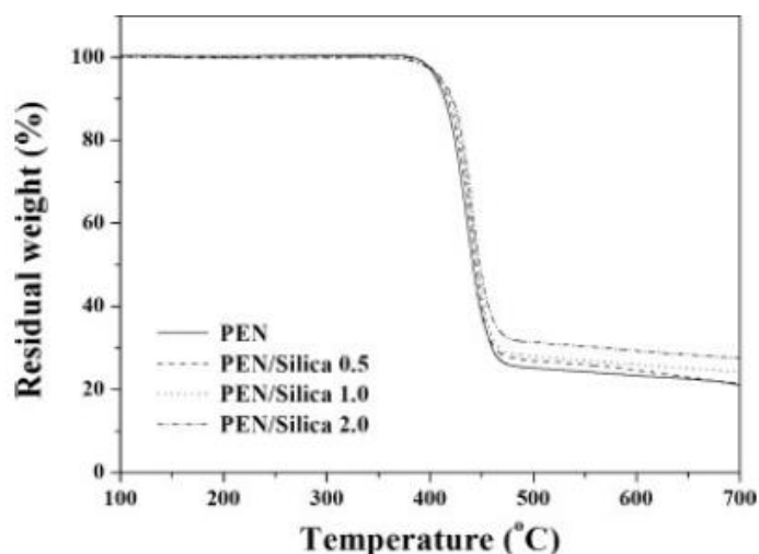
Slika 52. TG krivulje PEN/ \text{SiO}_2 nanokompozita s različitim sadržajem \text{SiO}_2 u struji dušika pri brzini zagrijavanja od 10\text{ }^\circ\text{C}/\text{min}
