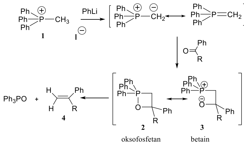
Shema 1. Mehanizam Wittigove reakcije.
