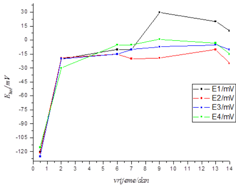
Slika 4-6: Ovisnost korozijskog potencijala o vremenu za leguru Cu-Ni pri temperaturi od 30°C
