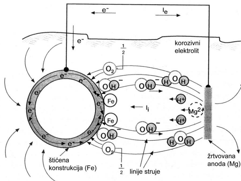
Slika 2-1: Shema katodne zaštite s galvanskom (žrtvovanom) anodom [5]
