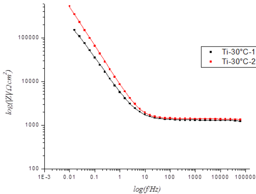
Slika 4-23: Ovisnost faznog kuta i logaritma apsolutne vrijednosti impedancije o logaritmu frekvencije za uzorak titana pri 30^\circ\text{C} ; točkama su prikazane izmjerene vrijednosti, a linijama vrijednosti izračunate prema modelu.
