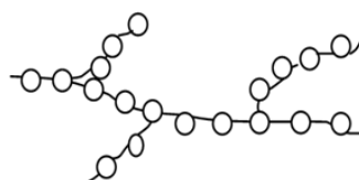
Slika 3. Granate makromolekule- shematski prikaz
