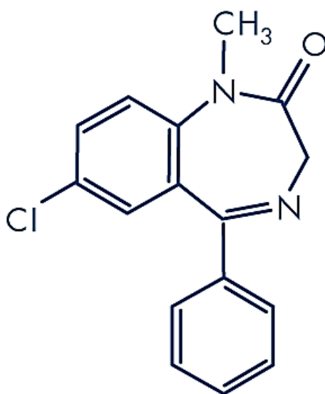
Slika 5. Strukturna formula diazepama
