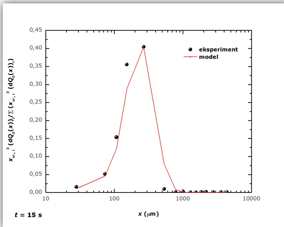
Slika 4.18. Usporedni prikaz simulirane i eksperimentalne raspodjele veličina čestica agrikulturne tvari; vrijeme granuliranja t = 15 s.
