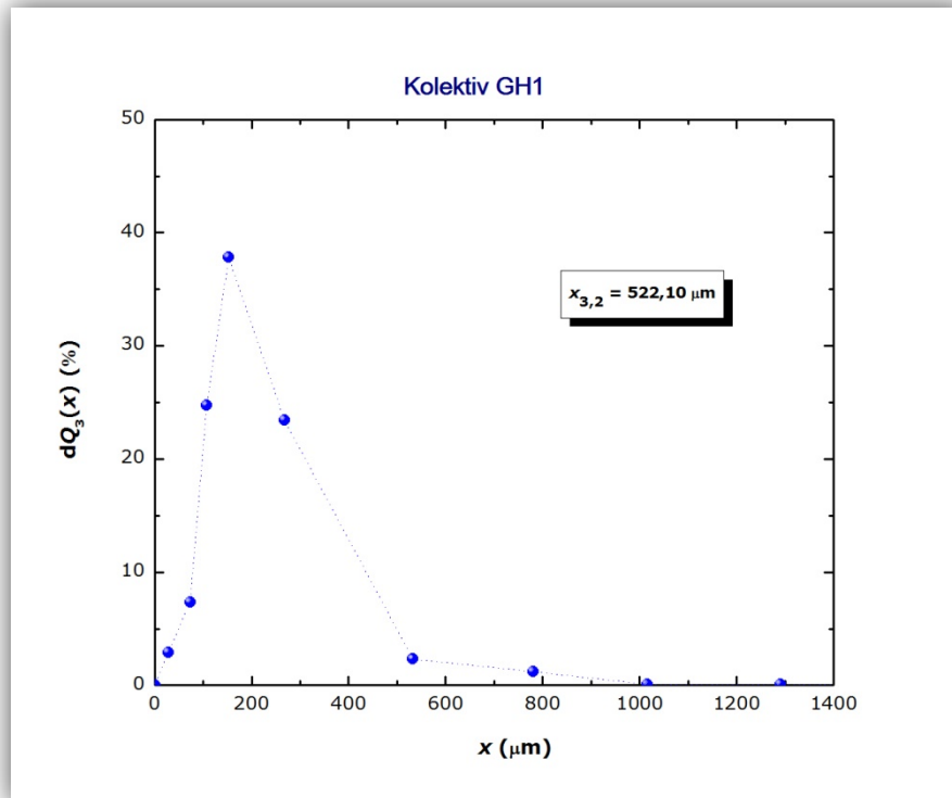
Slika 4.1. Grafički prikaz raspodjele veličina čestica Agrocal ® tvari u kolektivu GH1 dobivene analizom sitima.
