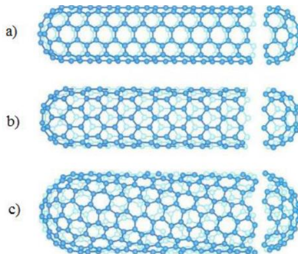
Slika 14. Različiti tipovi nanocjevčica s jednom stijenkom: a) akiralna – „fotelja“, b) akiralna – „cik cak“, c) kiralna
