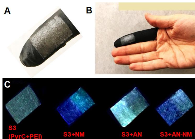
Slika 18. Nosivi nanovlaknasti senzor. A+B: nanovlaknasti dio nanesen na prst nitrilne rukavice. C: prenosivi senzor pokazuje velike promjene u boji u prisutnosti nitrometana, kao i u prisutnosti amonijevog nitrata i ANNAM. 53 (S3 – 1-pirenkarboskialdehid (PyrC) i polietilen imin (PEI))
