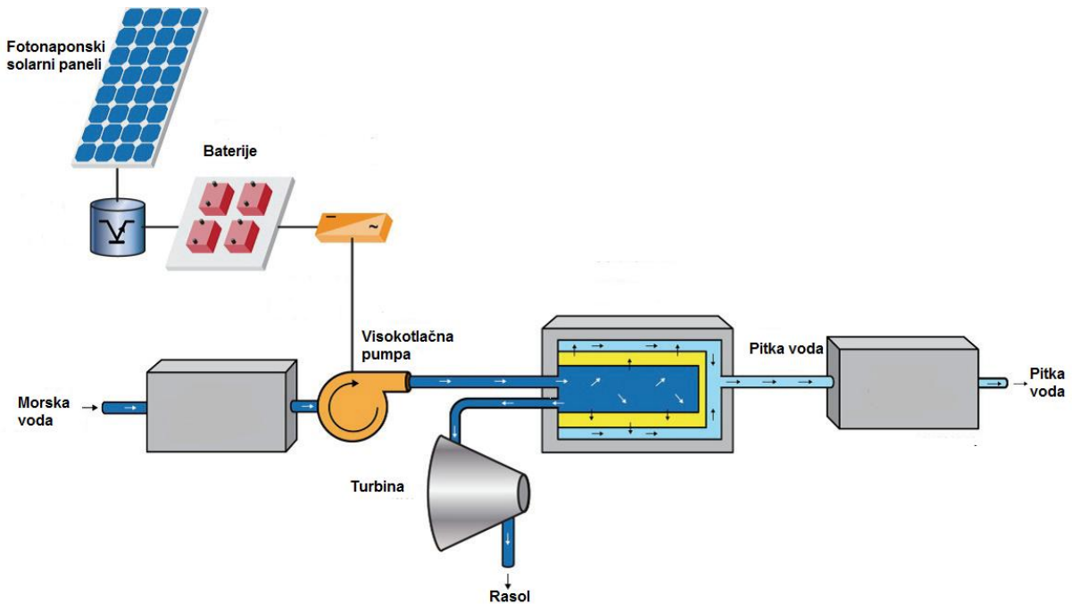
Slika 21. Shematski prikaz fotonaponskog sustava pokretanog sa reverznom osmozom [8].
