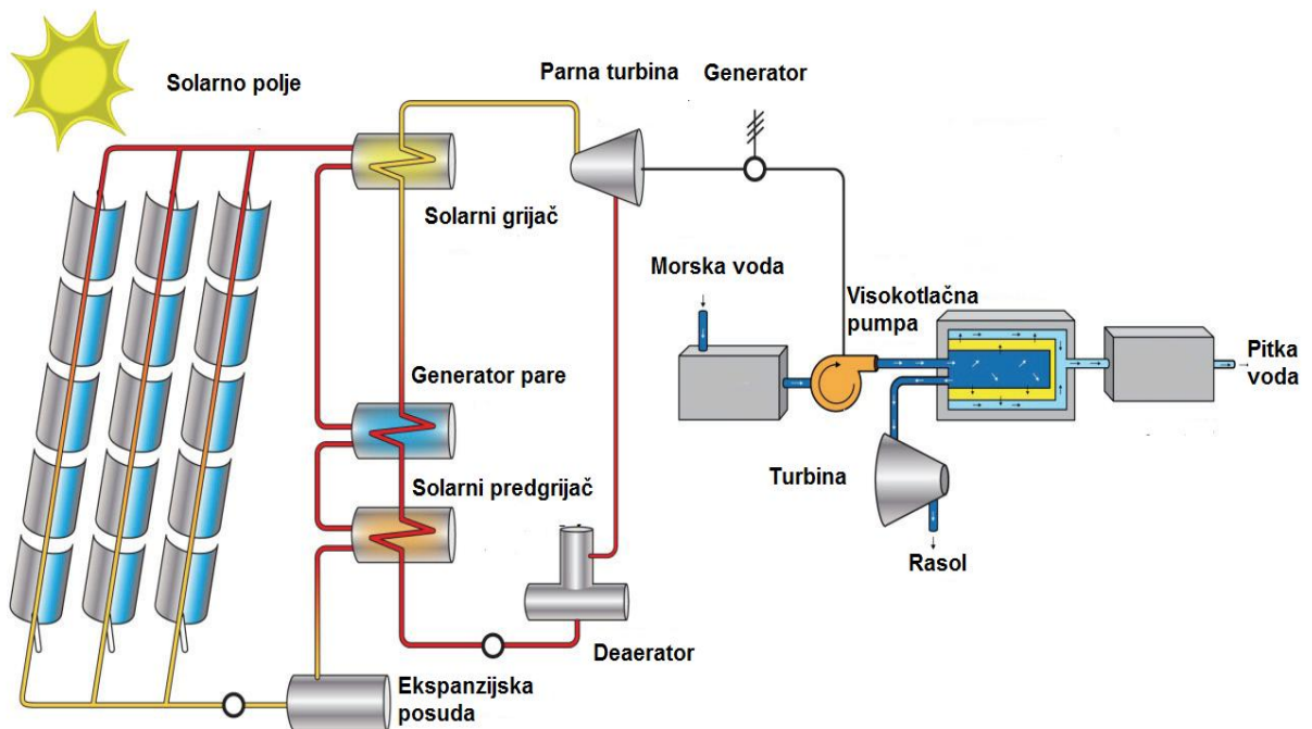
Slika 20. Shematski prikaz parabolnog korita u kombinaciji s RO postrojenjem [8].
