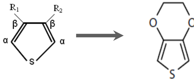
Slika 2.4. Prikaz sinteze 3,4-etilendioksitiofena iz tiofena
