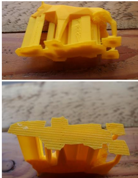
Slika 9. Prikaz 3D-tiskanog modela s opcijom raft
