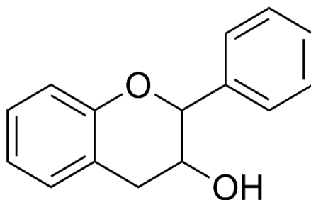
Slika 2.2. Monomer flavan-3-ol
