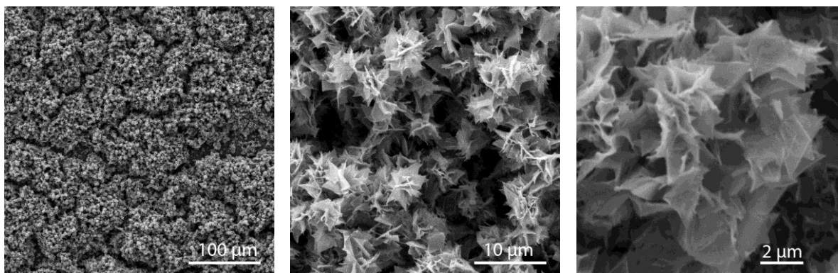
Slika 12. Prevlake dobivene iz otopine omjera 1:0:0,1 nakon 2 h sinteze i nakon žarenja na 300\text{ }^{\circ}\text{C}
