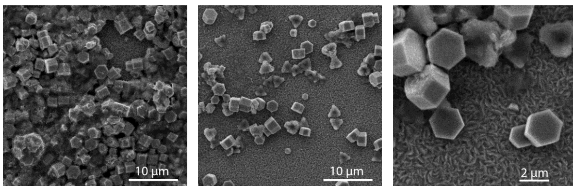
Slika 9. Prevlake dobivene iz otopine samog \text{ZnAc} \cdot 2\text{H}_2\text{O} nakon 4 h sinteze na 90^\circ\text{C} na podlogama sa slojem kristalnog sjemena
