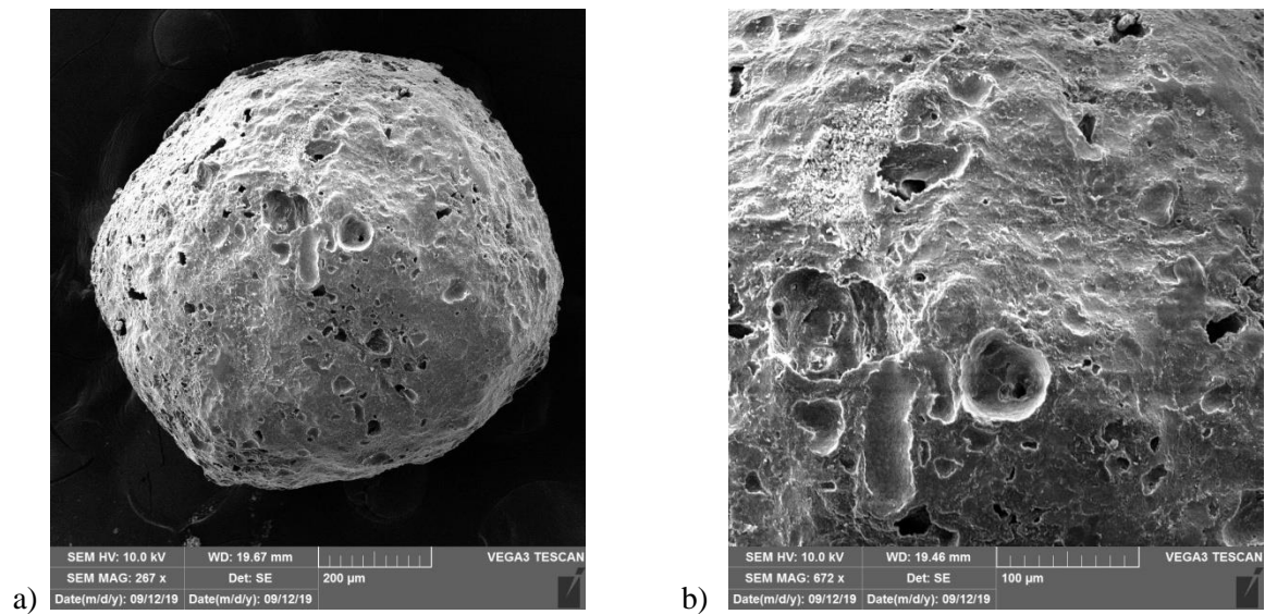
Slika 23. SEM-mikrografija: impregnirane pelete pri uvećanju: a) 200x; b) 500x
