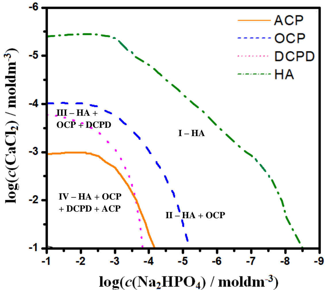
Slika 19. Granice taloženja ACP, OCP, DCPD i HA u sustavu \text{CaCl}_2 - \text{Na}_2\text{HPO}_4 , \text{pH} = 7,4 i t = 25 °C.
