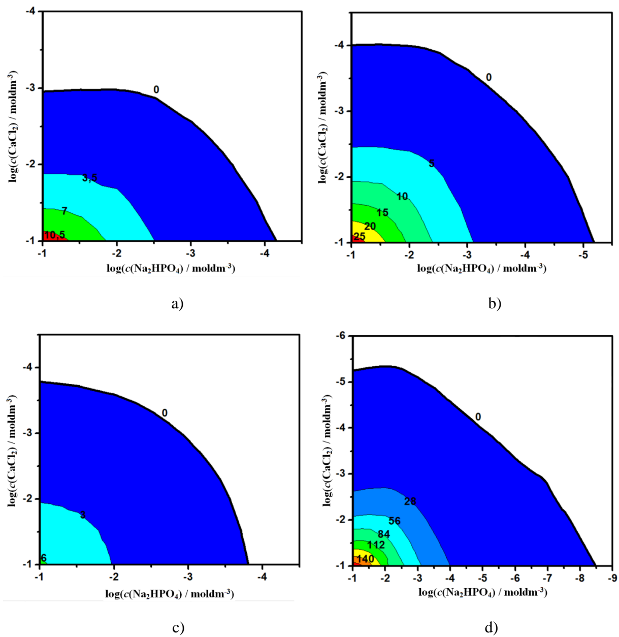
Slika 20. Taložni dijagrami: a) ACP-a, b) OCP-a, c) DCPD-a i d) HA u sustavu \text{CaCl}_2 - \text{Na}_2\text{HPO}_4 - \text{MgCl}_2 ( c = 0,0015 \text{ mol dm}^{-3} ), \text{pH} = 7,4 i t = 25^\circ\text{C} .
