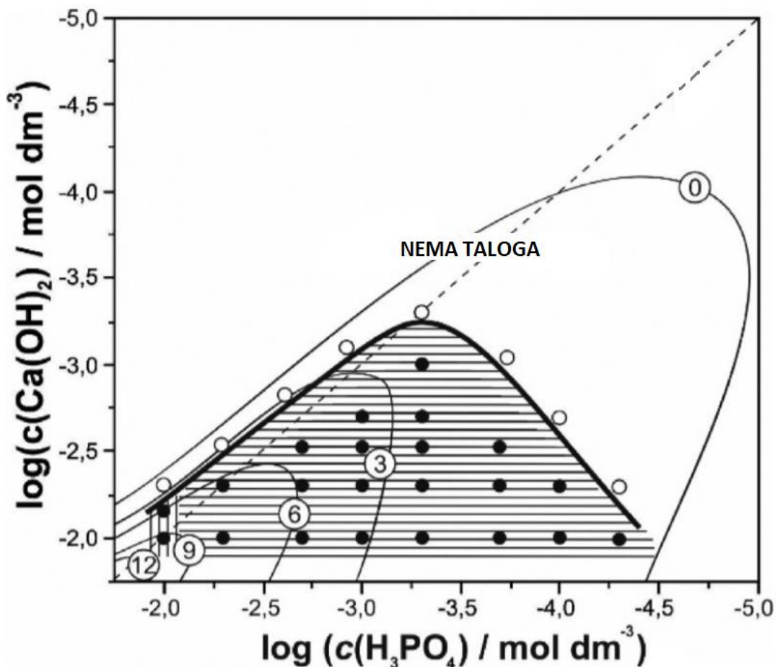
Slika 11. Taložni dijagram jednostavnog sustava, \text{Ca}(\text{OH})_2 - \text{H}_3\text{PO}_4 pri 25\text{ }^\circ\text{C} nakon 60 min starenja, \text{pH} = 2,2 - 12,3 . Konstruirano prema ref. 3.
