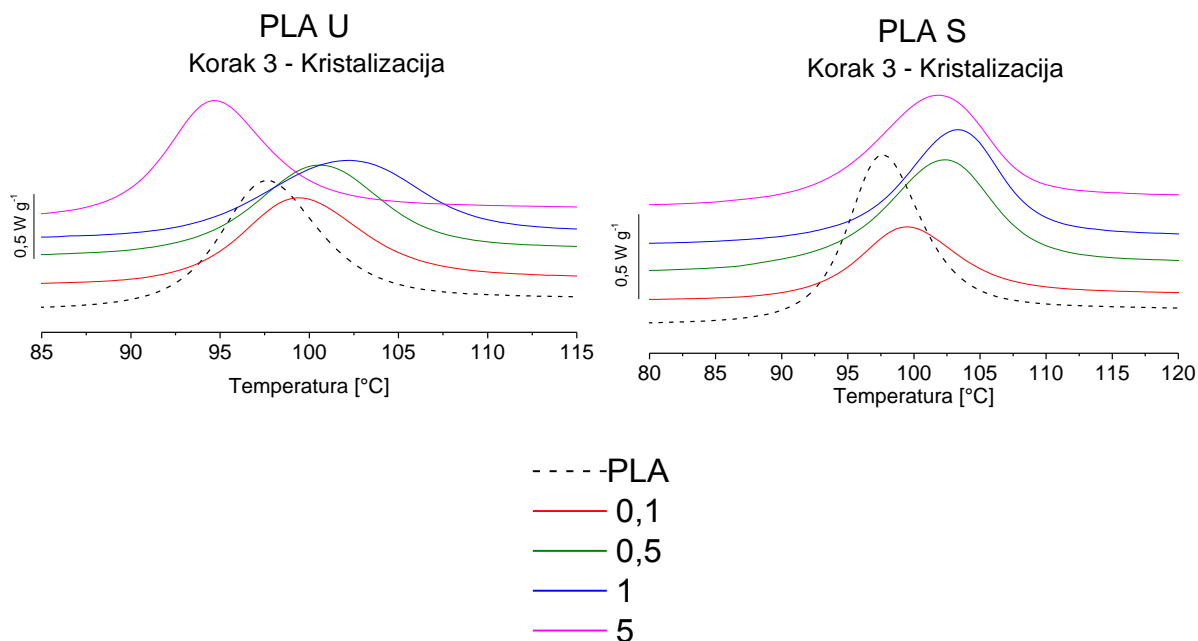
Slika 4.14. Kristalizacija za vrijeme prvog grijanja čistog PLA i kompozita sa Socal (S) i Solvay (U) punilima
