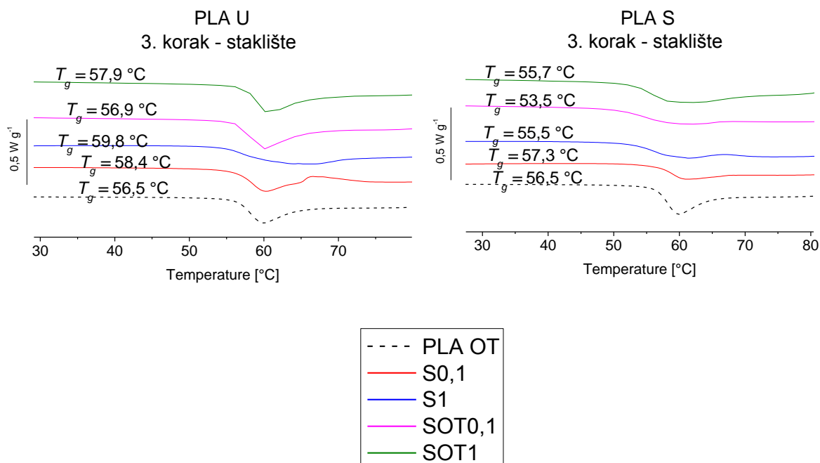
Slika 4.25. Staklište čistog PLA i kompozita sa Socal (S) i Solvay (U) punilom prilikom prvog grijanja
