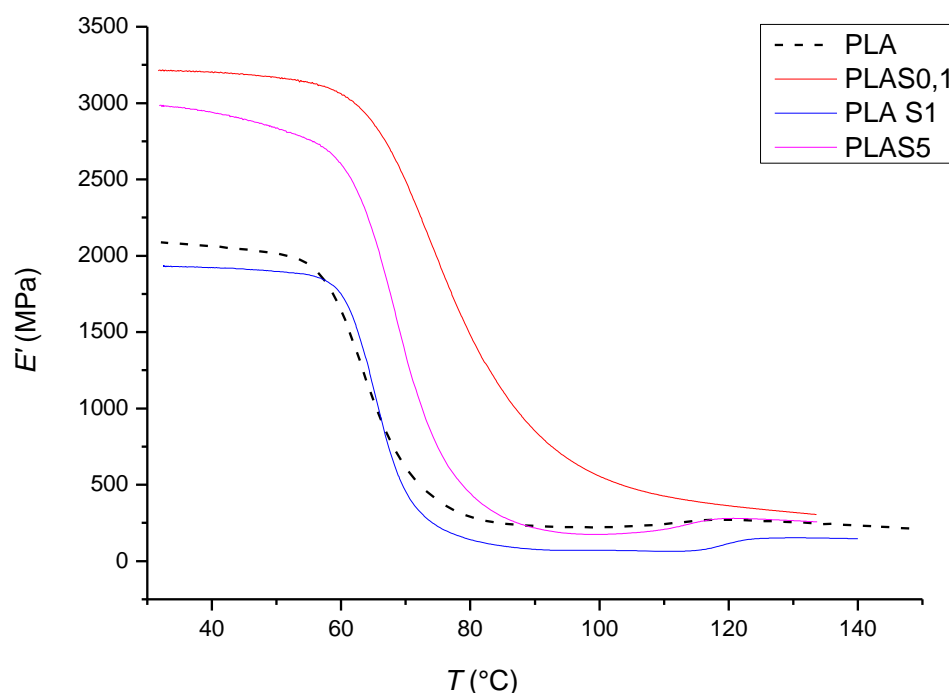
Slika 4.3. Ovisnost modula pohrane o temperaturi za PLA kompozite sa Solvol (S) punilom pripremljenih u Brabender gnjetalici
