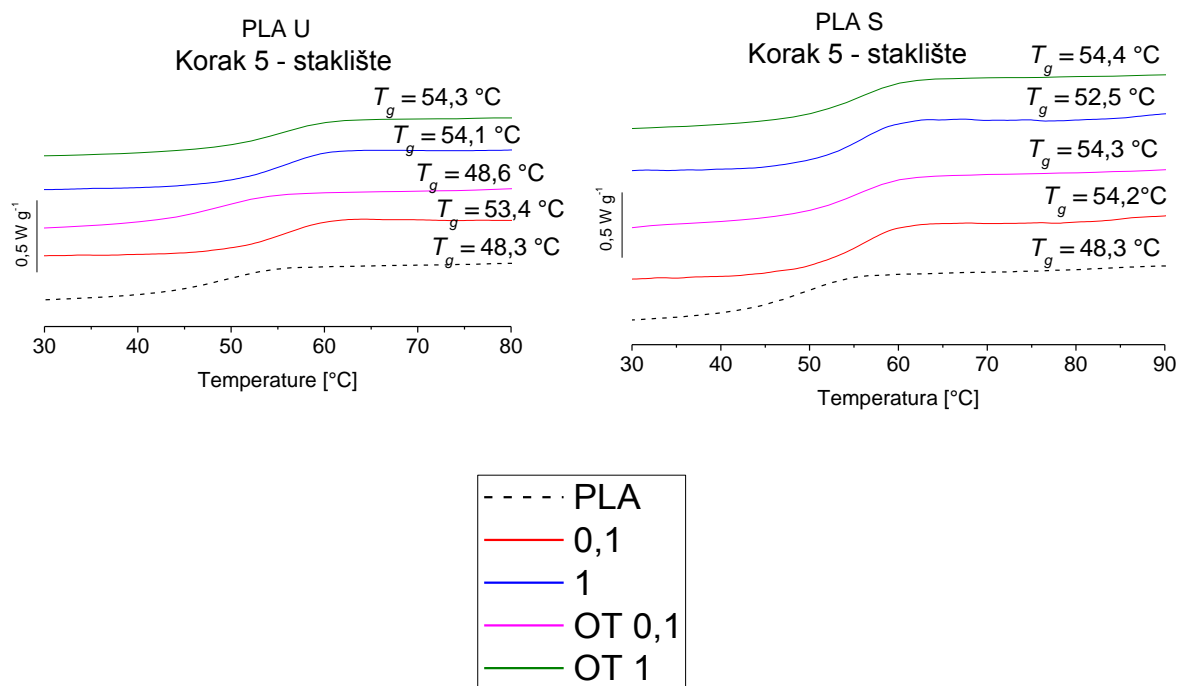
Slika 4.28. Staklište za vrijeme hlađenja čistog PLA iz otopine i kompozita sa Socal (S) i Solvay (U) punilom iz otopine i iz Brabender serije
