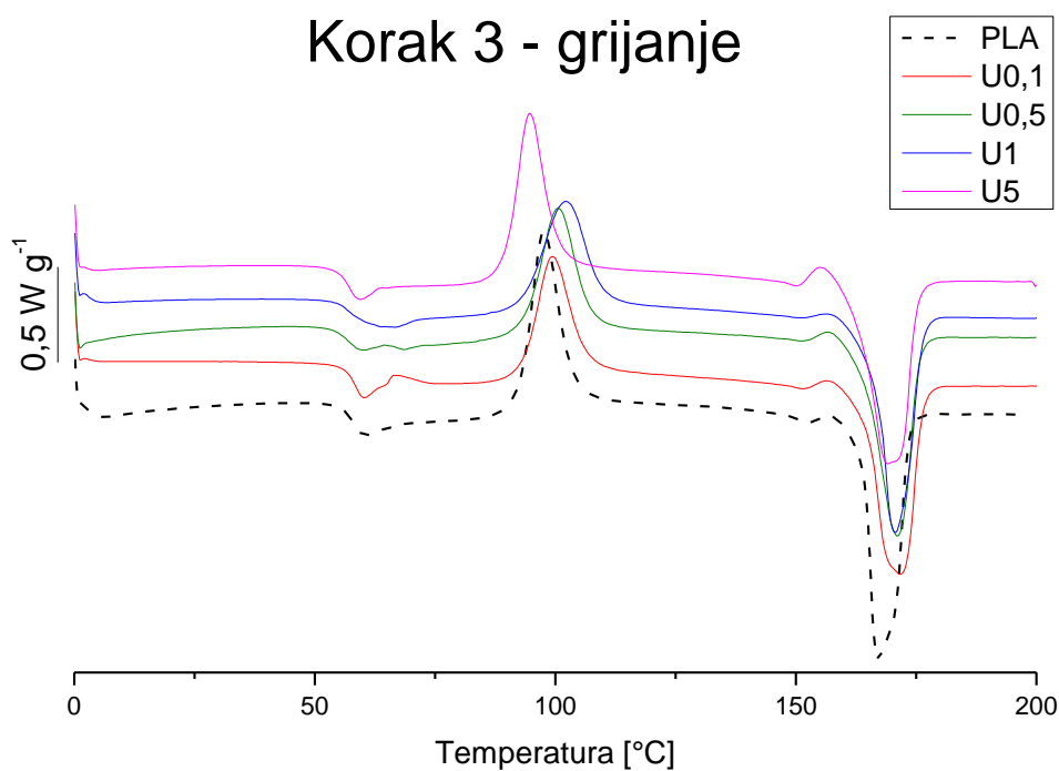
Slika 4.11. Treći korak DSC analize za kompozit sa Solvay (U) punilom iz Brabender serije
