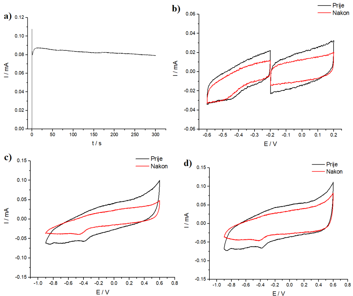
Slika 4.44. a) Strujni tranzijent zabilježen tijekom sinteze PEDOT/GO sloja na pozitivnoj elektrodi i ciklički voltamogrami zabilježeni za PEDOT/GO sloj, b) u užem području potencijala za pozitivnu elektrodu, c) u širem području potencijala za pozitivnu elektrodu i d) u širem području potencijala za negativnu elektrodu prije i nakon punjenja/pražnjenja superkondenzatora.
