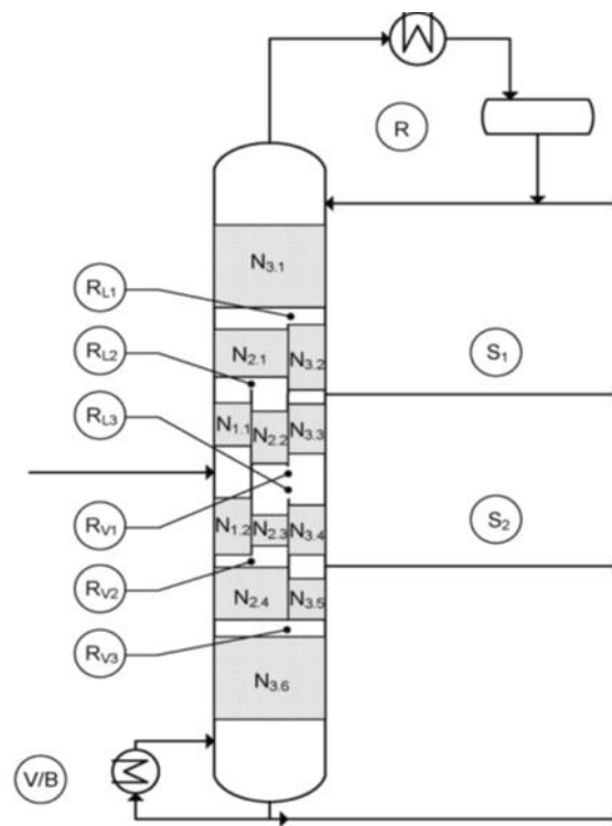
Slika 2.21. Petlyuk konfiguracija s razdjelnom stijenkom 13
