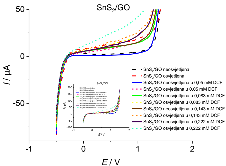
Slika 23. Voltamogram zabilježen za osvjetljenu i neosvijetljenu SnS 2 /GO elektrodu u 0,1 mol/dm 3 NaCl bez i s DCF u koncentracijama 0,05 mM, 0,083 mM, 0,143 mM i 0,222 mM.
