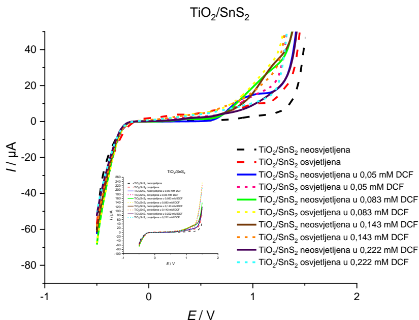
Slika 24. Voltamogram zabilježen za osvjetljenu i neosvijetljenu TiO 2 /SnS 2 elektrodu u 0,1 mol/dm 3 NaCl bez i s DCF u koncentracijama 0,05 mM, 0,083 mM, 0,143 mM i 0,222 mM.
