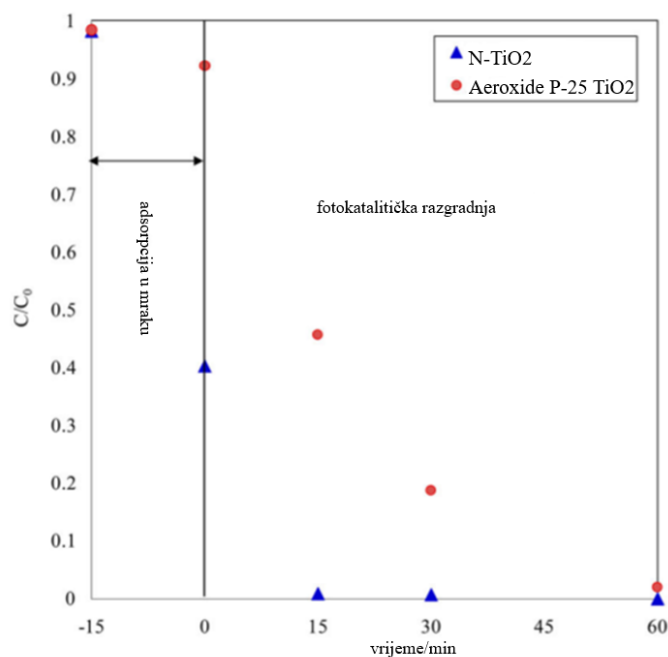
Slika 3.16. Usporedba učinkovitosti fotokatalizatora za fotokatalitičku razgradnju CFX-a [93].
