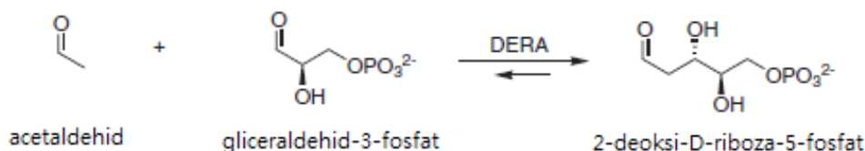
Slika 3. Konverzija 2-deoksi-D-riboze-5-fosfata, in vivo reakcija katalizirana DERA-om. 9
