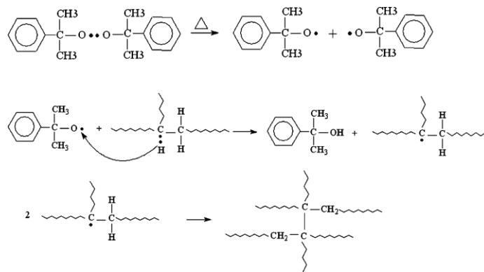
Slika 10. Kemijske reakcije umrežavanja polietilena upotrebom dikumil peroksida kao katalizatora umrežavanja [25].
