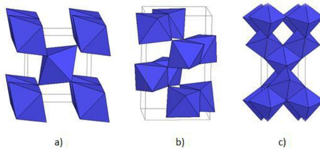
Slika 2.2.1. Kristalne modifikacije TiO 2 : a) rutil, b) bruakit, c) anatas
