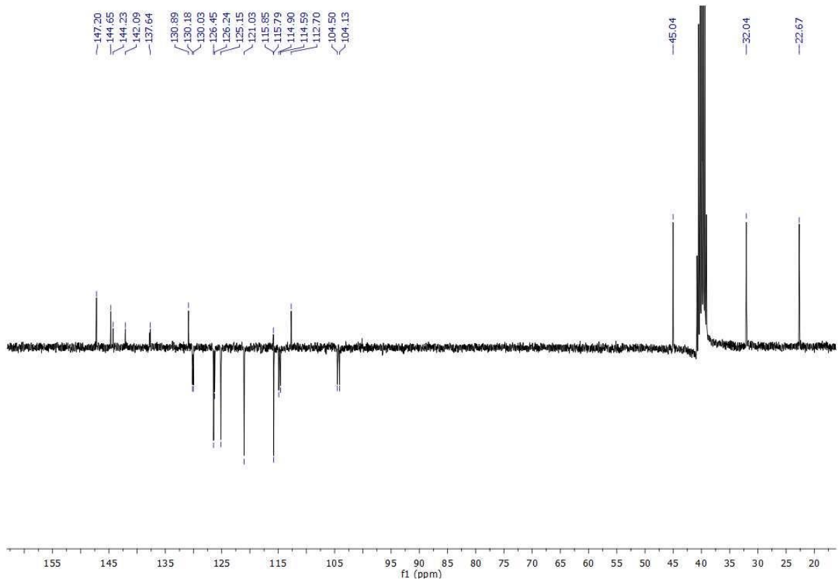
Slika 27. 13 C NMR spektar spoja 18
