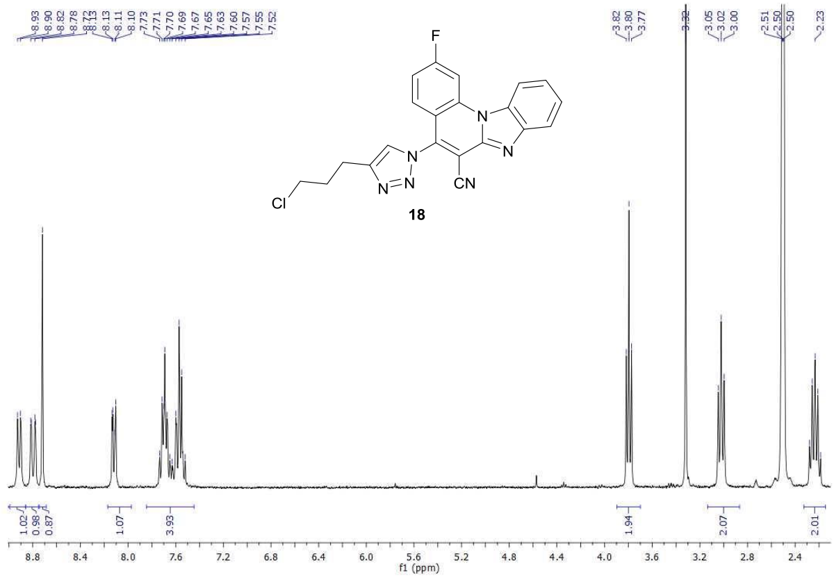
Slika 26. 1 H NMR spektar spoja 18
