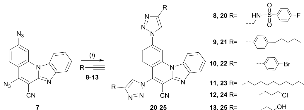
Shema 18. Sinteza bis-1,2,3-triazolilnih derivata benzimidazo[1,2-a]kinolin-6-karbonitrila ( 20–25 ). Reagensi i uvjeti: (i) Cu(OAc) 2 ·H 2 O, metanol
