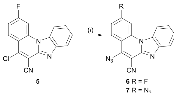
Shema 14. Sinteza monoazidnog derivata 6 i diazidnog derivata 7. Reagensi i uvjeti: (i) NaN 3 , aceton
