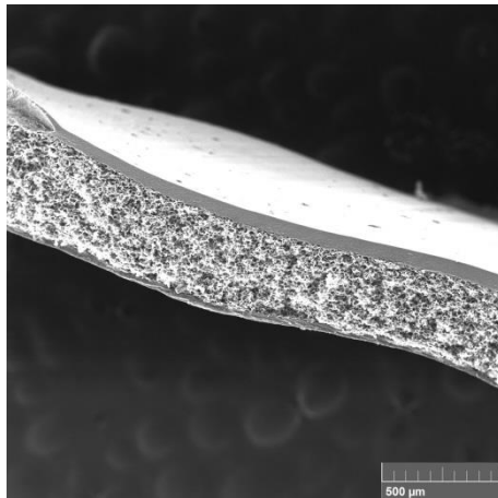
Slika 5.10. SEM mikrograf uzorka 5-G-HG
