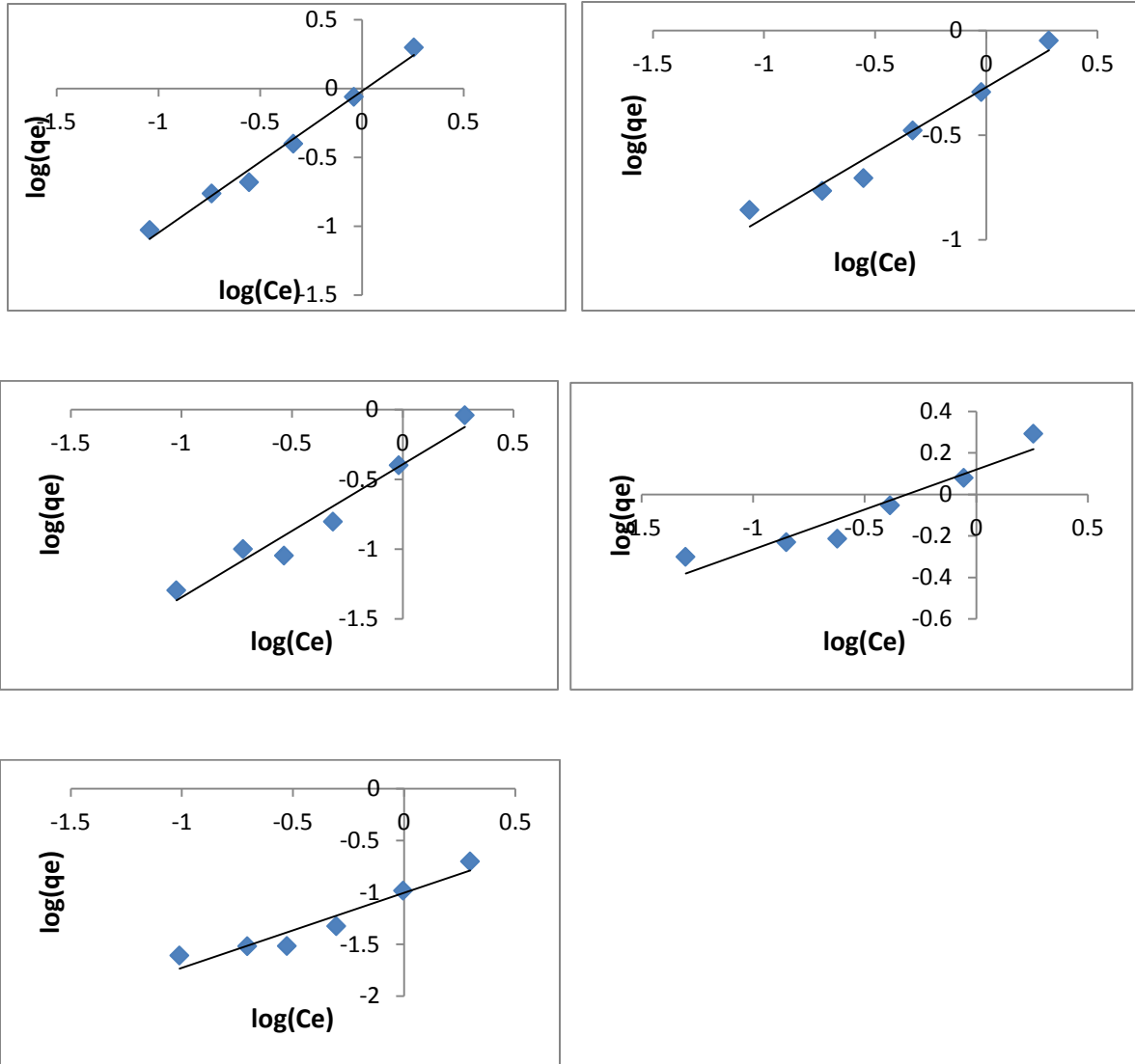
Slika 4.3.3. Linearzirane Freundlichove sorpcijske izoterme (s lijeva na desno) za sedimente Glina, Lonja, Pakra, Petrinjčica i Studena za otopinu pripremljenu s 0,01 M \text{CaCl}_2
