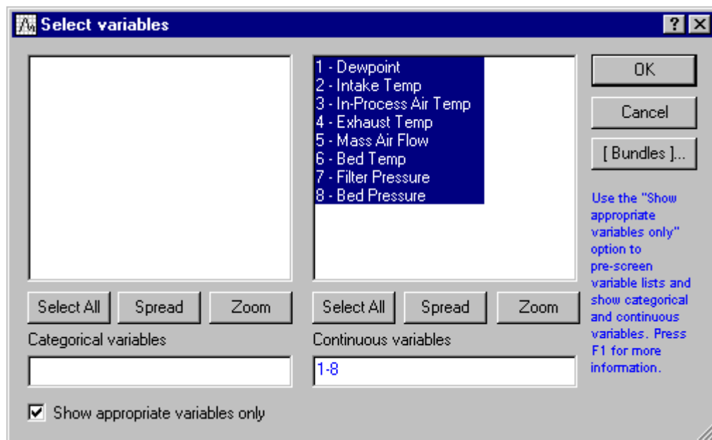
Slika 9. Odabir varijabli
