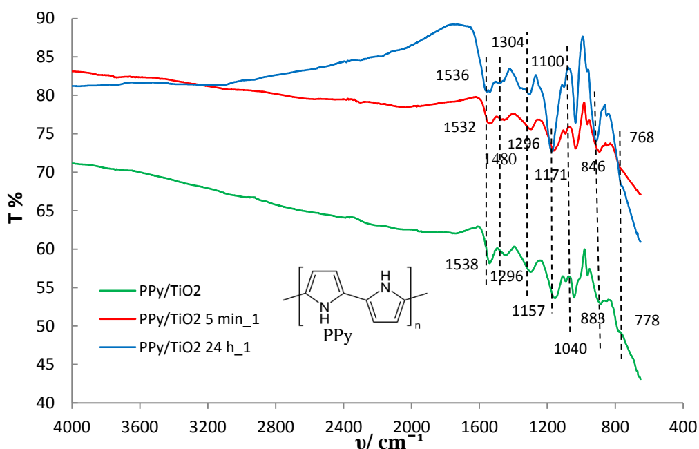
Slika 4.1. FTIR spektri nedomificiranog i PPy/TiO 2 fotokatalizatora deprotoniranih s 0,1M NH 4 OH u vremenu od 5 min i 24 sata, serija PPy/TiO 2 -1
