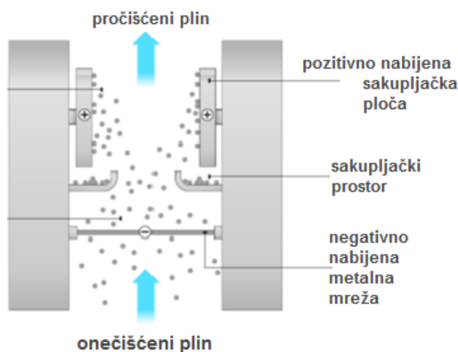
Slika 14. Shema jednostavnog elektrofiltra [44]
