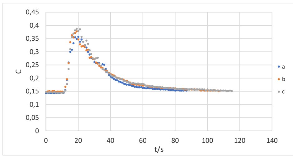
Slika 3.4. Ponovljeni eksperiment za 1. cijev za volumen 0,3 ml i protok od 201 ml/min
