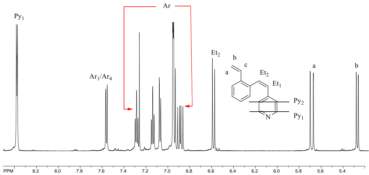
Slika 9. ^1\text{H} NMR spektar cis-2 .
