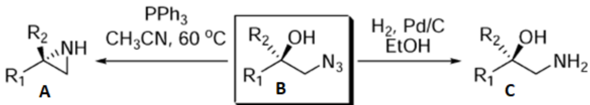
Slika 2.9. Proizvodnja azirdina (A) i aminoalkohola (C) redukcijom iz azidoalkohola (B) dobivenog biotehnološkom putem s HHDH 92
