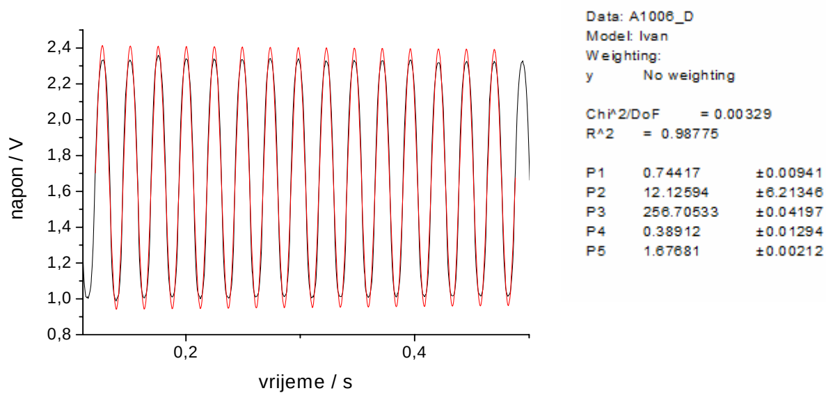
Slika 4. g) Određivanje rezonantne frekvencije uzorka debljine 10mm
