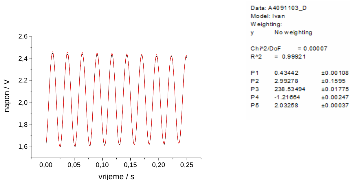
Slika 4. d) Određivanje rezonantne frekvencije uzorka debljine 4mm
