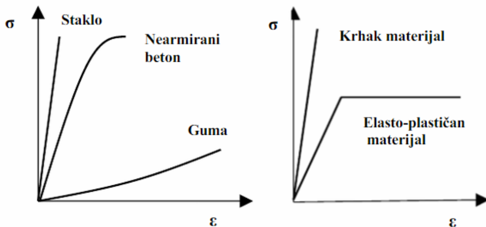
Slika 1.c) Ovisnost naprezanja o istezanju krhkih i elastičnih materijala
