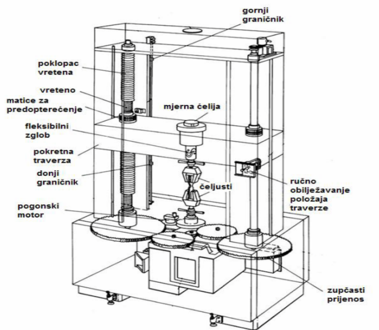
Slika 2.a) Shema kidalice (10)
