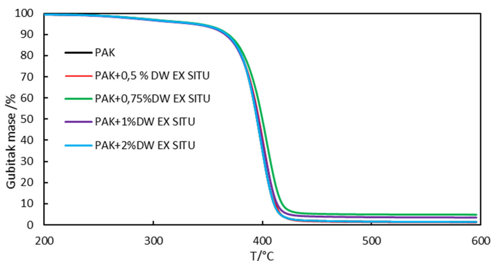
Slika 77. TGA krivulja PAK i PAK/TiO 2 ex situ premaza.
