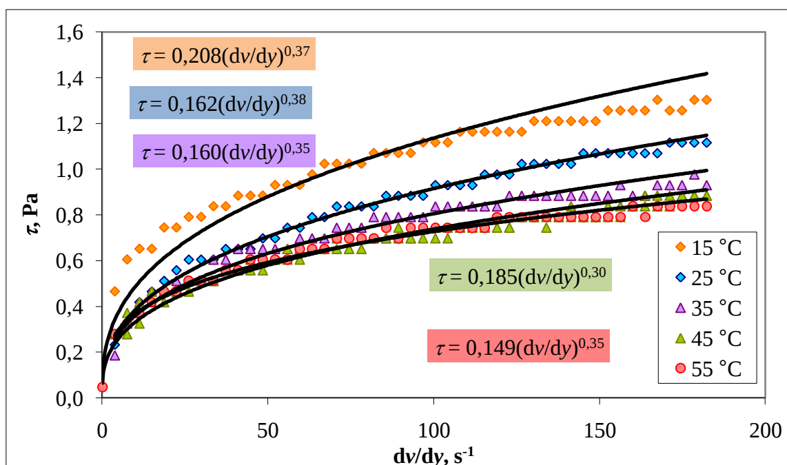
Slika 23. Promjena smičnog napreznja sa smičnom brzinom –za 1M uzorak s dodatkom SDS (0.1 mas%).
