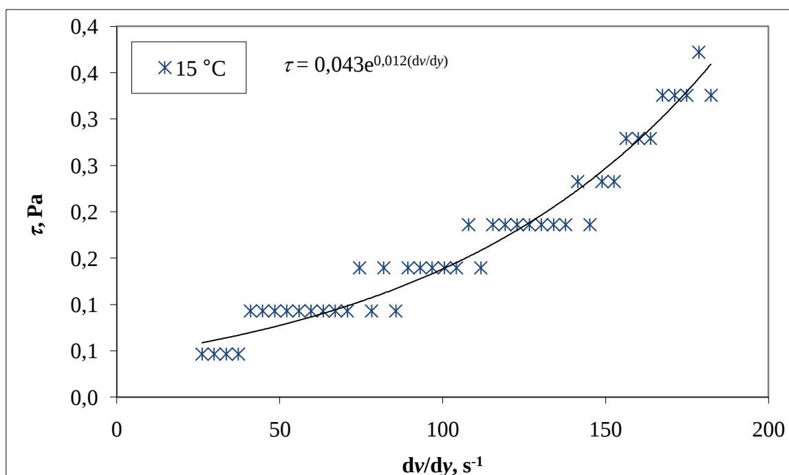
Slika 21. Promjena smičnog naprezanja sa smičnom brzinom –za 1M uzorak s dodatkom CTAB (0.0132 mas%) za 15 °C.
