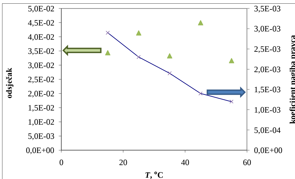
Slika 20. Ovisnost nagiba i odsjeka aproksimacijskog pravca sa temperaturom.
