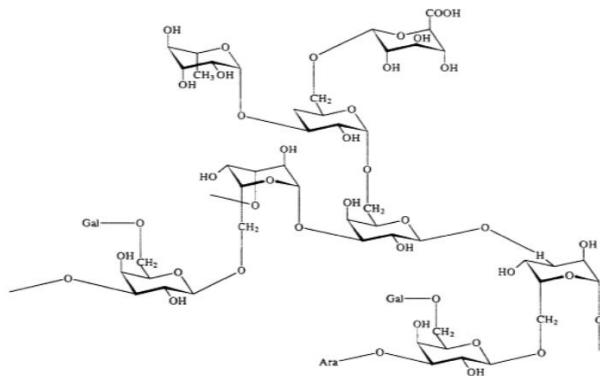
Slika 8. Strukturna formula arapske gume
