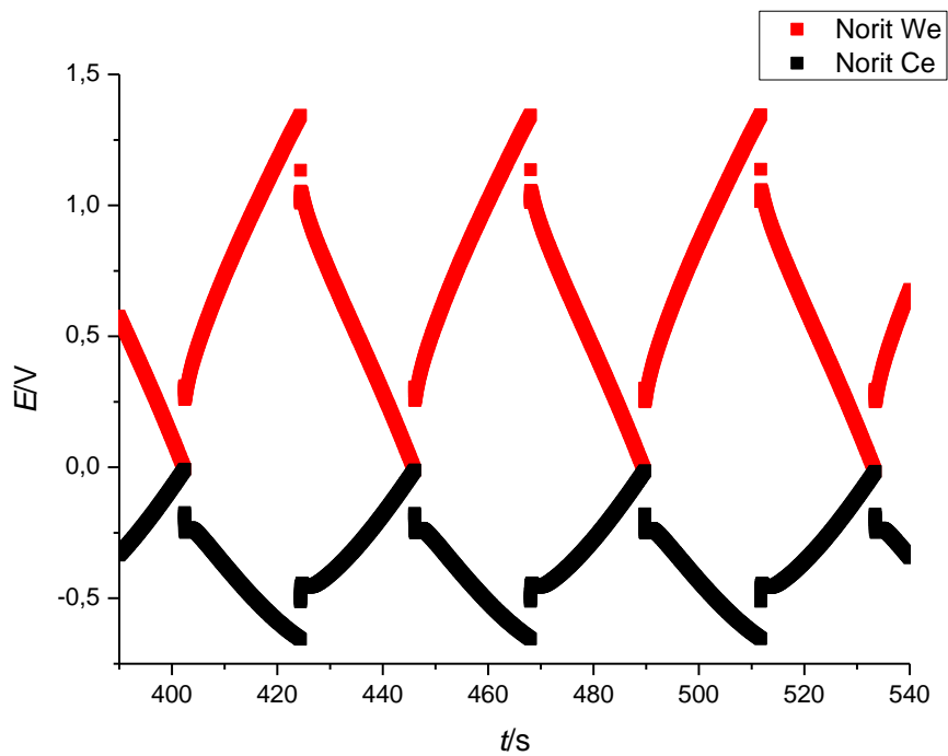
Slika 35. Tri ciklusa punjenja/praznjenja strujom od 20 mA za za materijal Norit u troelektrodom sustavu
