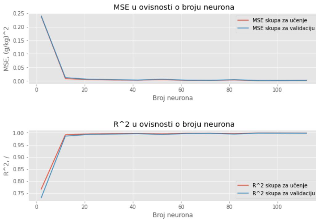
Slika 4.2. MSE i R^2 u ovisnosti o broju neurona za sigmoid aktivacijsku funkciju
