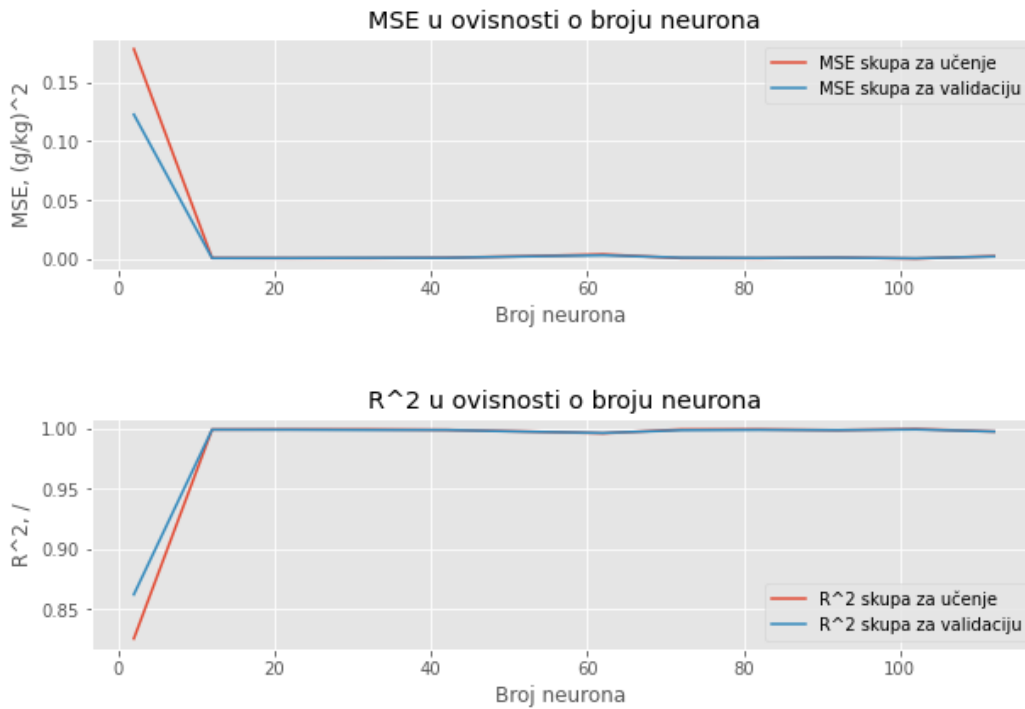
Slika 4.1. MSE i R^2 u ovisnosti o broju neurona za ReLU aktivacijsku funkciju
