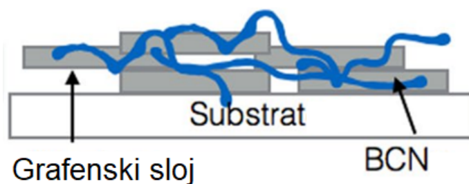
Slika 2.1 Shematski prikaz GN/BCN senzora.
