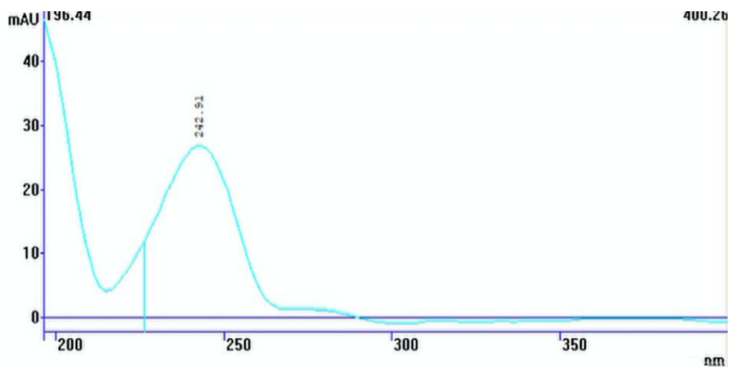
Slika 20. ApSORpcijski spekatar razgradnog/transformacijskog produkta FEB u retentatu s vremenom zadržavanja t_R = 23,558 min
