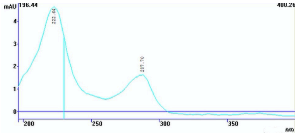
Slika 14. Apсорpcijski spekтар razgradnog/transformacijskog produkta FEB u permeatu s vremenom zadržavanja t_R = 17,347 min
