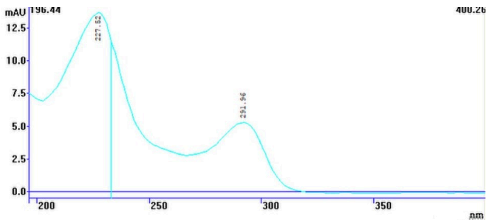
Slika 15. Apсорpcijski spekтар razgradnog/transformacijskog produkta FEB u permeatu s vremenom zadržavanja t_R = 21,211 min
