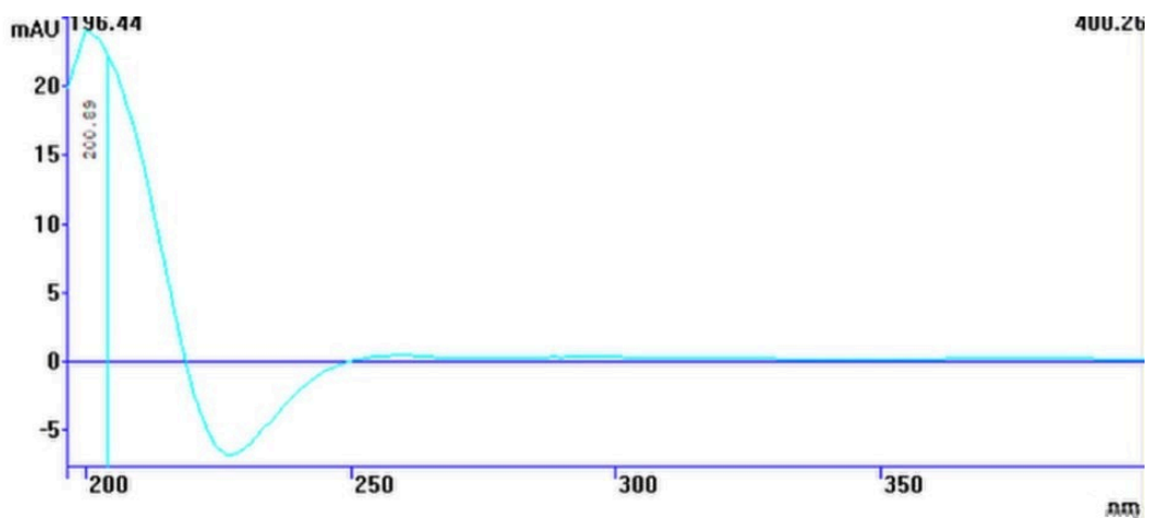
Slika 18. Apсорpcijski spekter razgradnog/transformacijskog produkta FEB u retentatu s vremenom zadržavanja t_R = 5,198 min
