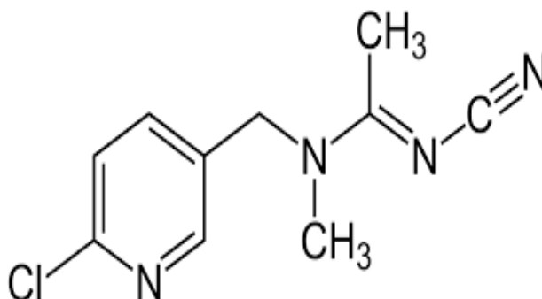
Slika 4. Strukturna formula acetamiprida [20]
