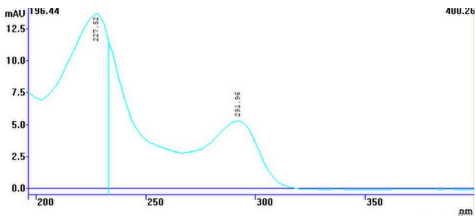
Slika 15. ApSORPCIJSKI SPECTAR RAZGRADNOG/TRANSFORMACIJSKOG PRODUKTA FEB U PERMEATU S VREMENOM ZADRŽAVANJA t_R = 21,211 min
