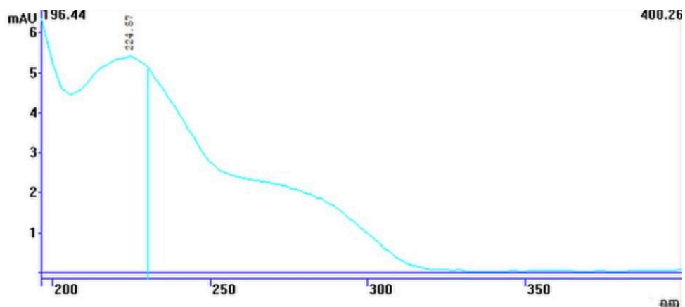
Slika 16. ApSORPCIJSKI SPECTAR RAZGRADNOG/TRANSFORMACIJSKOG PRODUKTA FEB U PERMEATU S VREMENOM ZADRŽAVANJA t_R = 23,1730 min
