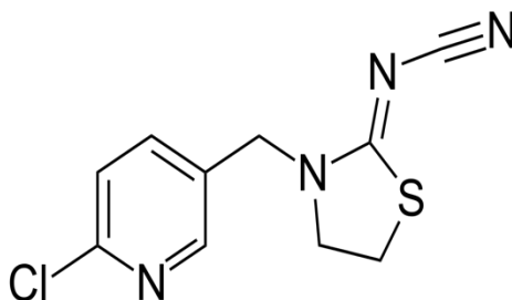
Slika 5. Strukturna formula tiakloprida [21]
