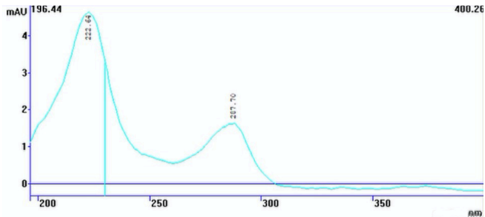
Slika 14. ApSORPCIJSKI SPECTAR RAZGRADNOG/TRANSFORMACIJSKOG PRODUKTA FEB U PERMEATU S VREMENOM ZADRŽAVANJA t_R = 17,347 min
