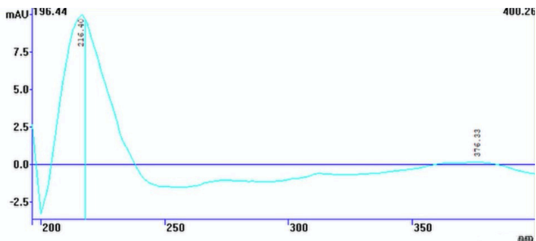
Slika 19. ApSORPCIJSKI SPEKTAR RAZGRADNOG/TRANSFORMACIJSKOG PRODUKTA FEB U RETENTATU S VREMENOM ZADRŽAVANJA t_R = 21,607 min
