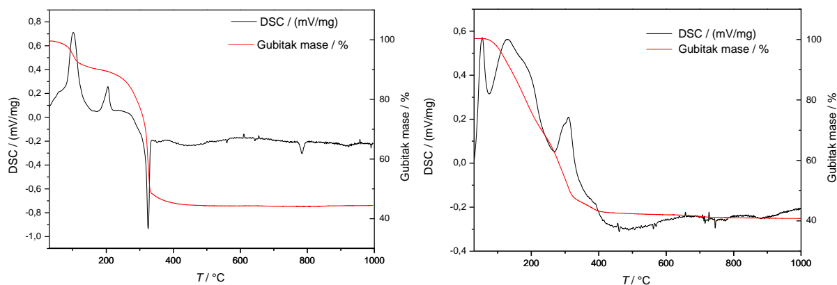
Slika 23. DTA/TGA grafovi uzoraka s 0 mol.% Co pripremljenih s cink (II) nitratom ( ZCxN (lijevo) i ZCxNn (desno))
