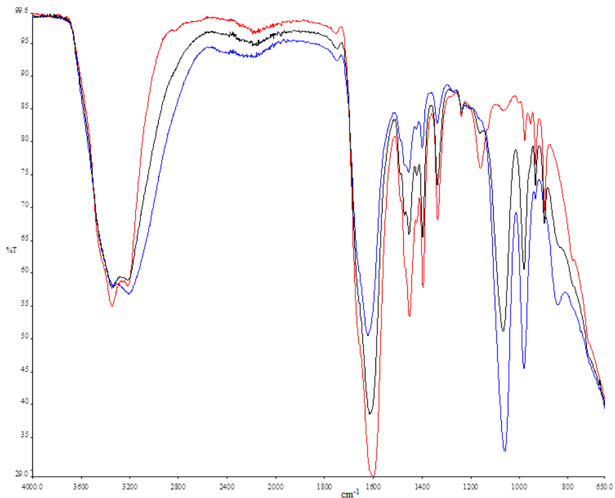
Slika 8. Rezultati FTIR analize za DES B:U (1:3) 40% (— čisti DES, — uzorak enzima nakon šaržne ekstrakcije s DES pri koncentraciji K 2 HPO 4 od 0,8 g/mL, — uzorak nakon šaržne ekstrakcije s DES pri koncentraciji K 2 HPO 4 od 0,9 g/mL)
