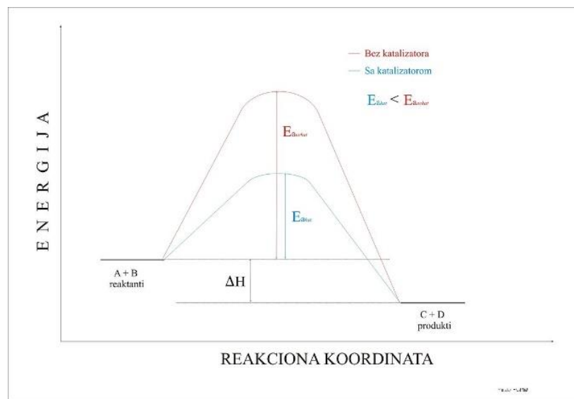
Slika 2.1. Mehanizam katalize
